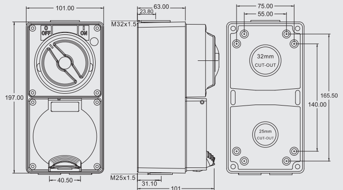
外形尺寸 Dimension
