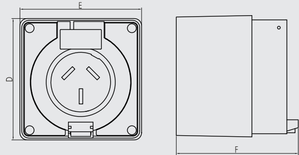
外形尺寸 Dimension
