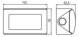
插座 Socket 16A-250V~ 表面安装 IP55 Surface mount
