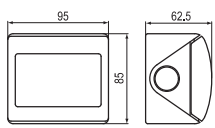
4联开关 4 Gang switch 13A-250V~ 表面安装 IP55 Surface mount
