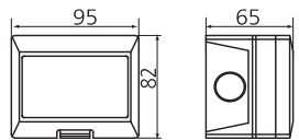
插座 Socket 13A-250V~ 表面安装 IP55 Surface mount
