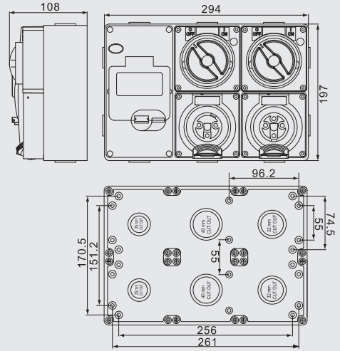
外形尺寸 Dimension
