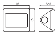
开关插座 Switch socket 15A-250V~ 表面安装 IP55 Surface mount
