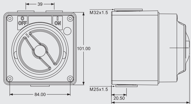
外形尺寸 Dimension
