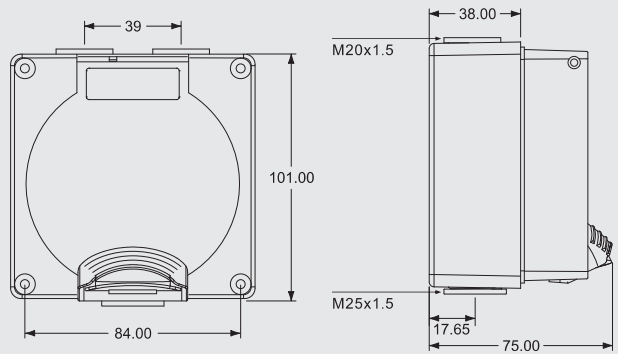
外形尺寸 Dimension
