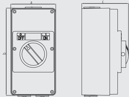
外形尺寸 Dimension
