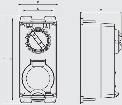
外形尺寸 Dimension
