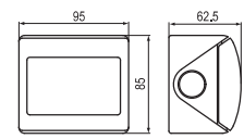
开关插座 Switch socket 13A-250V~ 表面安装 IP55 Surface mount
